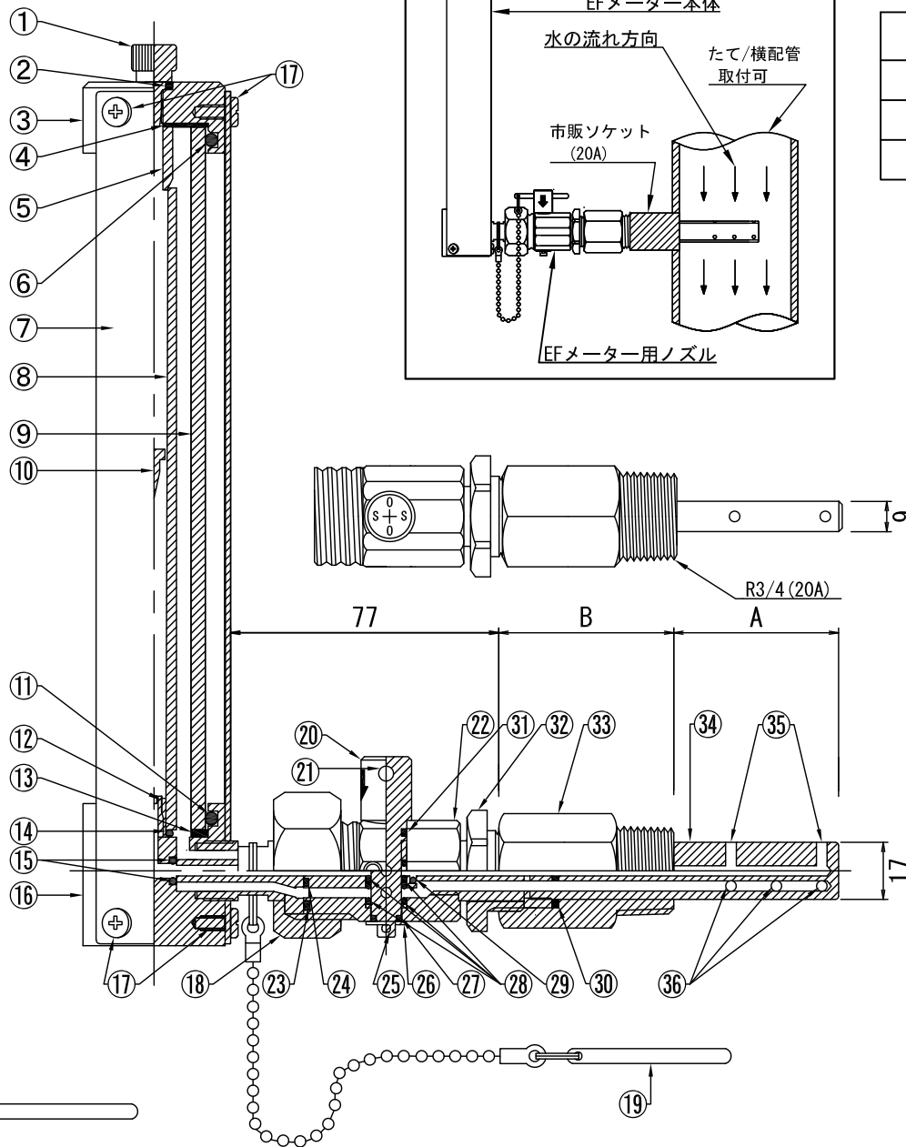
型式別流量表及びピトー管(A)/ユニオンネジ(B)寸法
